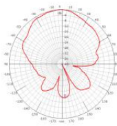
2690MHz
