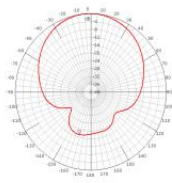
698MHz
